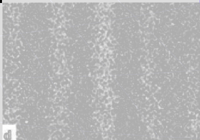
Franges linéaires d'électrons
